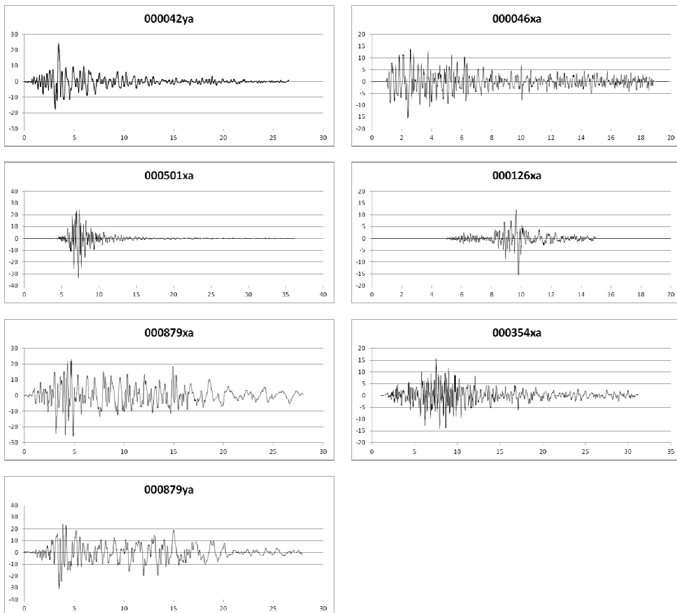
Fig. 11: Accelerogrammi non scalati dei 7 sismi di riferimento.
